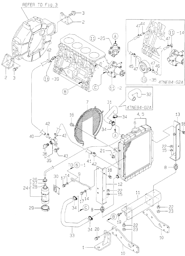
Fig.12. RADIATOR
